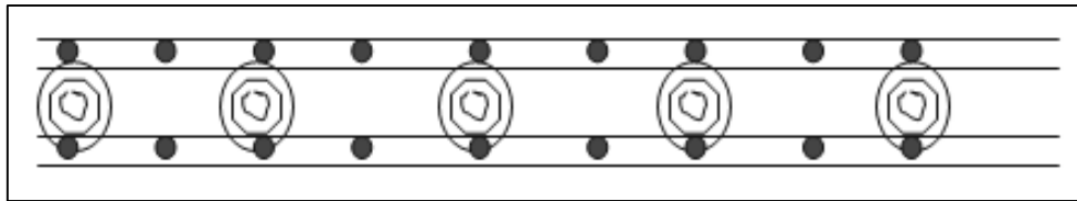
Figura 4.4. Esquema de goteros en franjas
